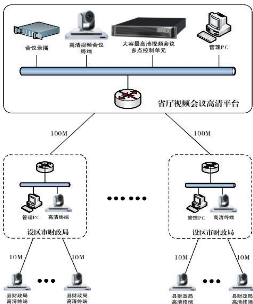
全省财政高清视频会议系统架构图
